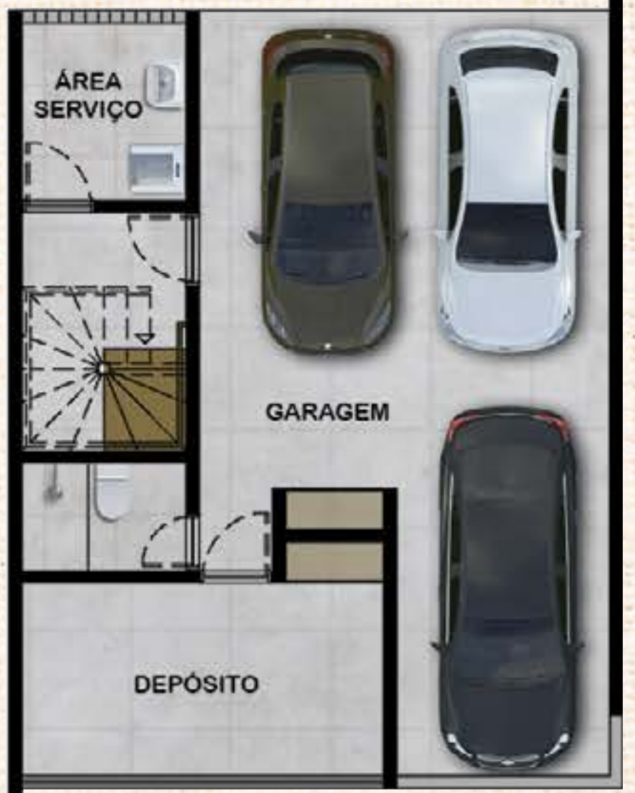
PAVIMENTO SEMIENTERRADO
