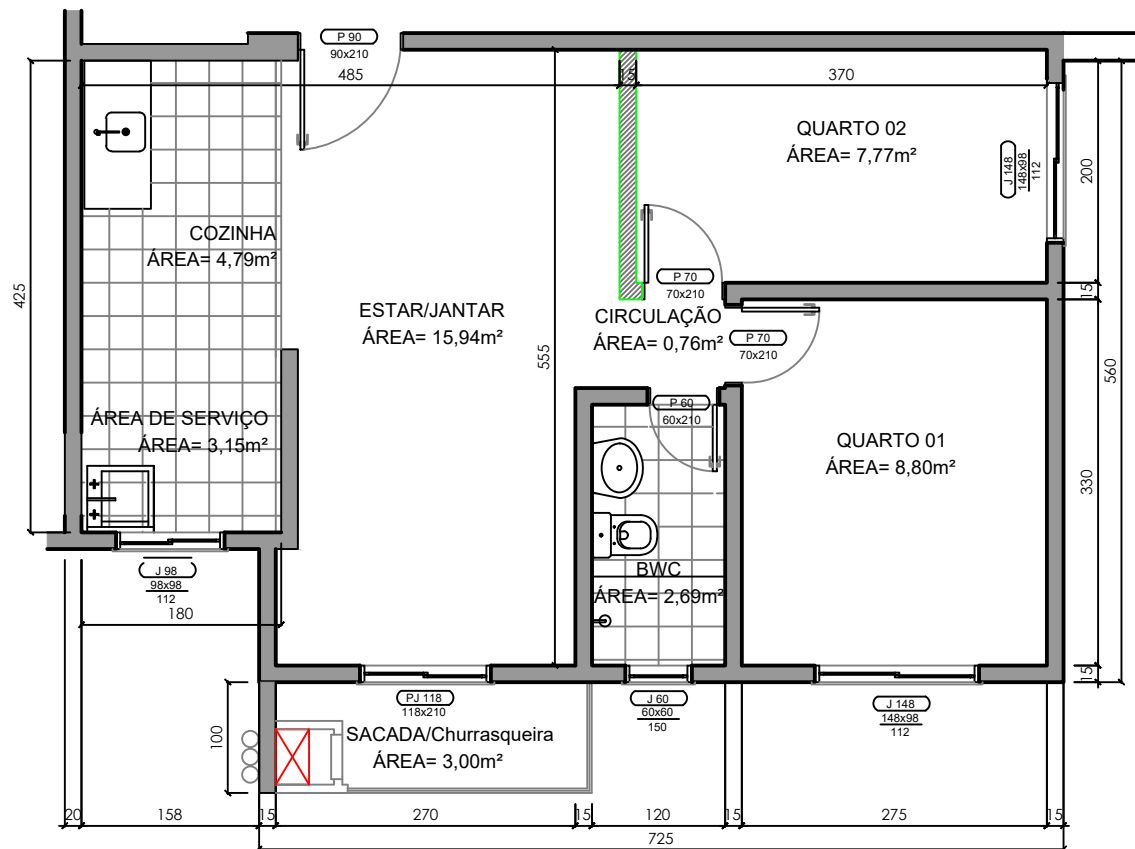
APARTAMENTO 2 QUARTOS PAVIMENTO SUPERIOR ÁREA= 52,53 m 2 ESCALA 1:60
