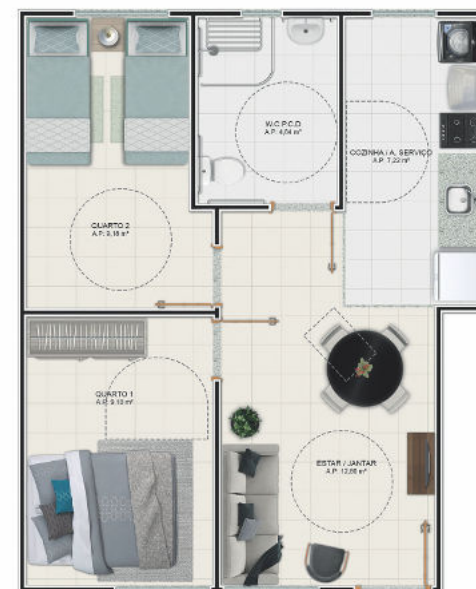
Planta Humanizada Und. Habitacional Tipo Adaptado
