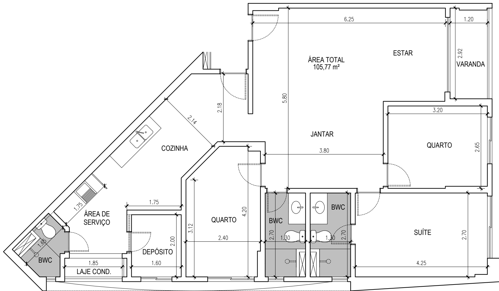
PLANTA BAIXA 3 QUARTOS TERMINADOS EM 01 - TIPO - TORRES A e B ESC. _____/175
