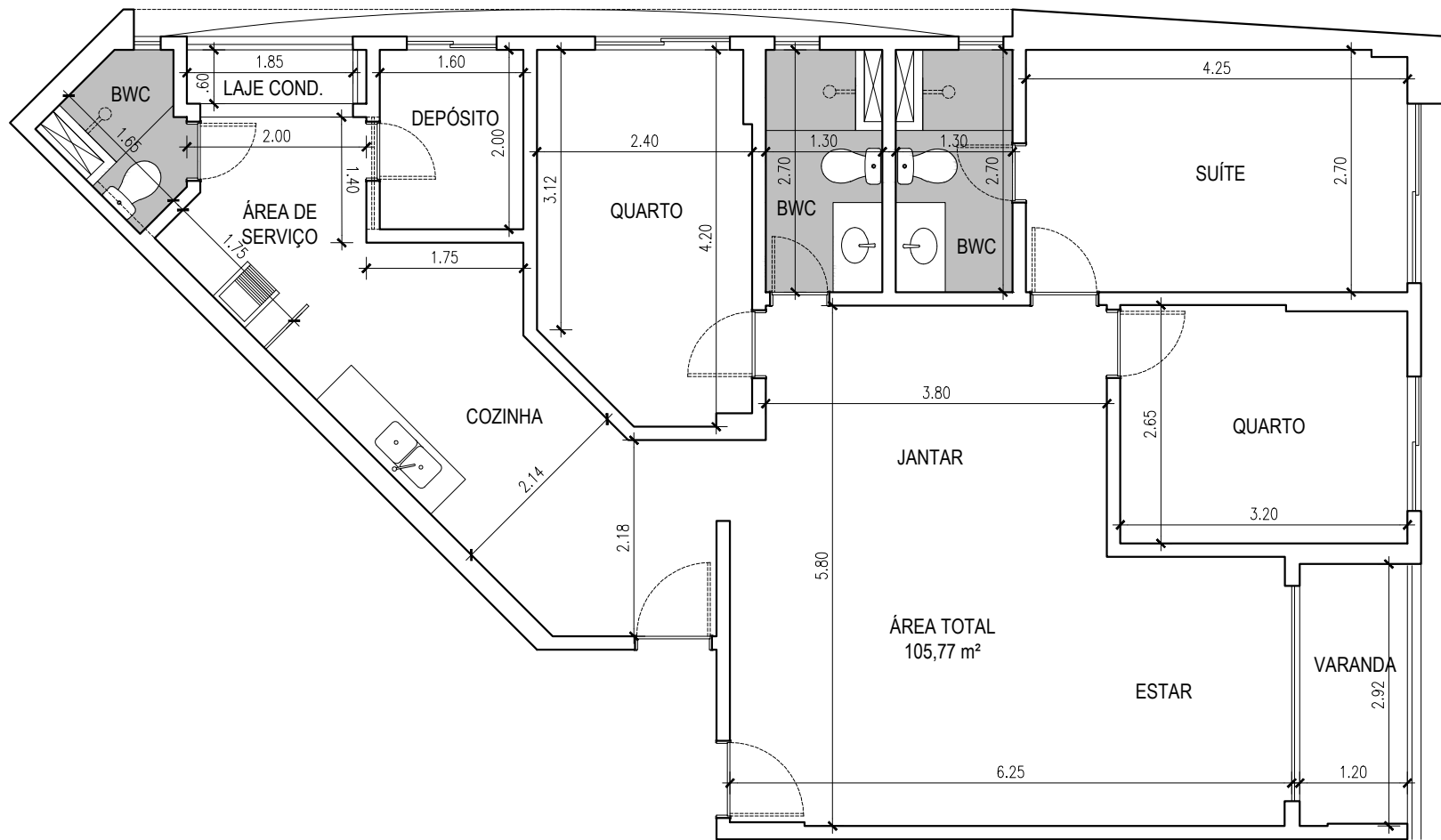
PLANTA BAIXA 3 QUARTOS TERMINADOS EM 03 - TIPO - TORRES A e B ESC. _____/175
